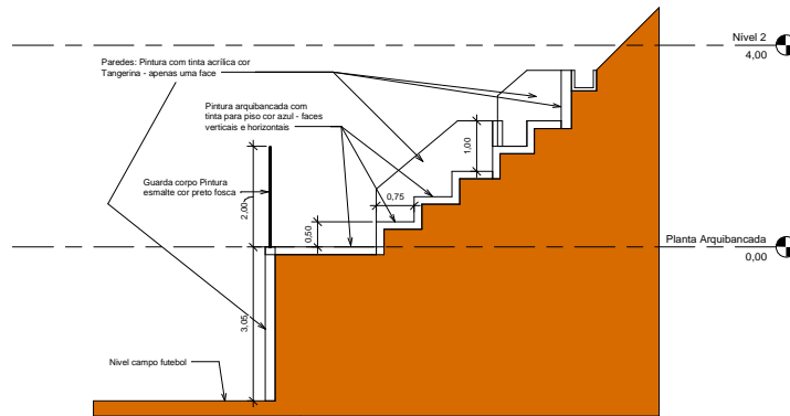
2 Corte 1 1 : 50
