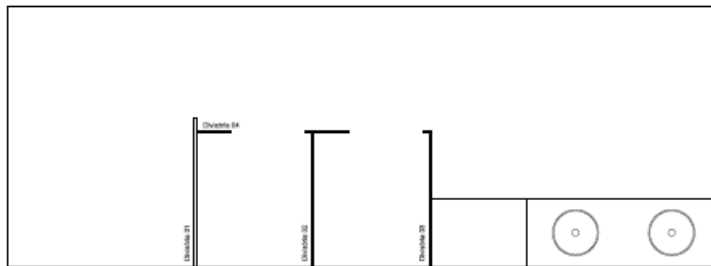
WC Feminino - Croqui esquemático Escala: 1/25
