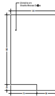
WC Feminino - Vista Divisória 01 Escala: 1/25
