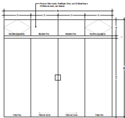
Porta 02 - Tipo de Correr: 04 unidades Escala: 1/25
