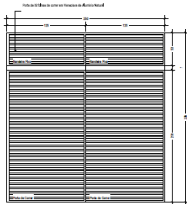
Porta 05 - Tipo de Correr: 01 unidade Escala: 1/25
