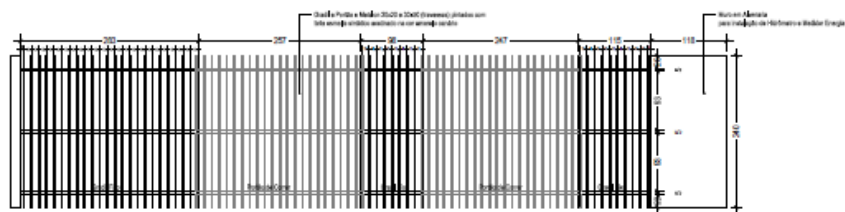
Grade/Fôrdo Frontal - Tipo de corer Escala: 1/50
