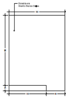
WC Masculino - Vista Divisória 05 Escala: 1/25
