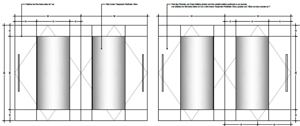
Porta 01 - Tipo Pivoteante: 04 unidades de 180x290 Escala: 1:25
