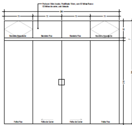
Porta 02 - Tipo de Correr: 04 unidades Escala: 1/25
