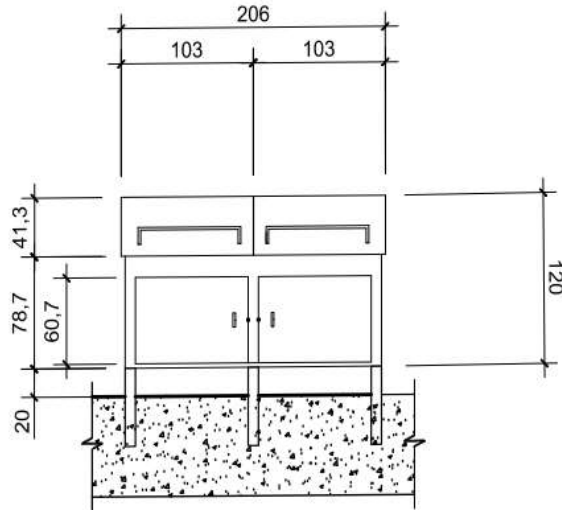
01 Vista Frontal Lixeira Roça
