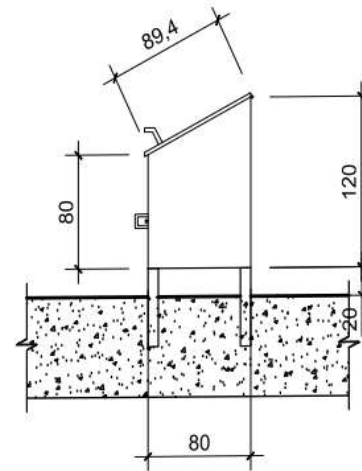
02 Vista Lateral Lixeira Roça
